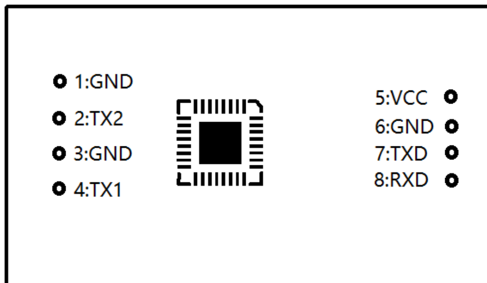
图 1: 接口示意图
